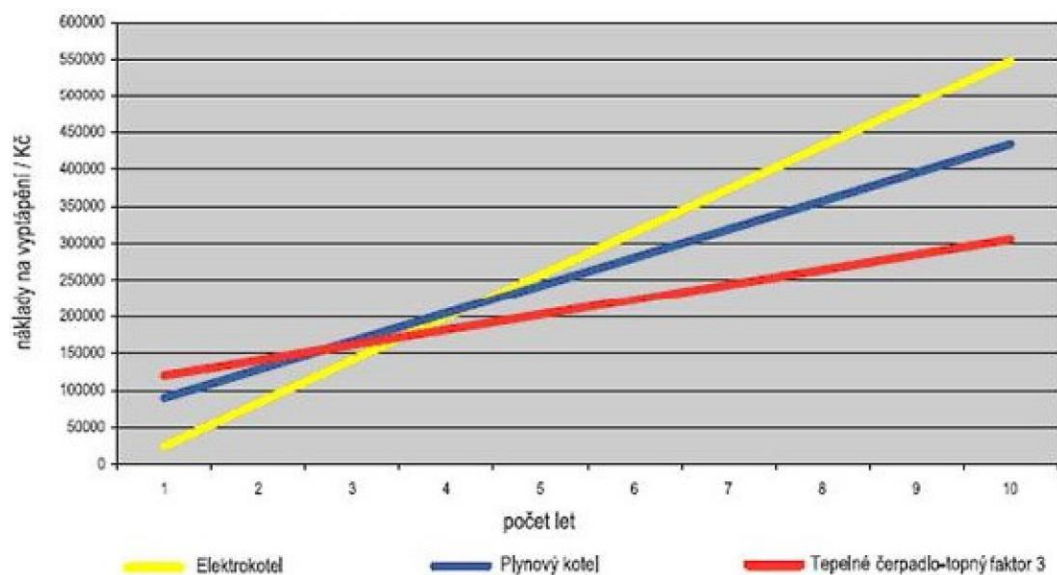
Obr. 4: Graf návratnosti investice u vytápění středního domu (spotřeba 3000 kWh, ohřev 200 TUV/den, dvoukanálová topná soustava). TUV – teplá užitková voda.
