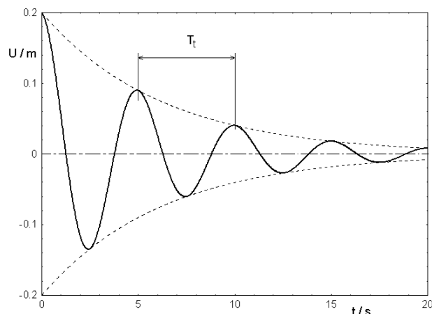
obr. 6.2 Časový průběh výchylky tlumených kmitů.
