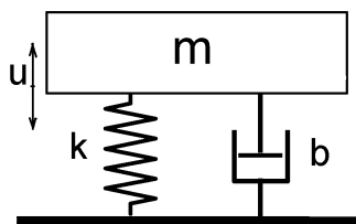
obr. 6.1 Schéma tlumené mechanické soustavy.
