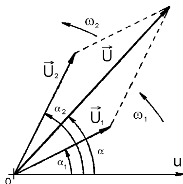
obr. 8.2 Fázorový diagram
