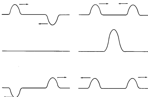
obr. 11.2 Šíření vlnění – vlevo destruktivní, vpravo konstruktivní
