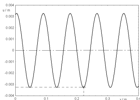
obr. 9.14 Vlna v čase 18 s
