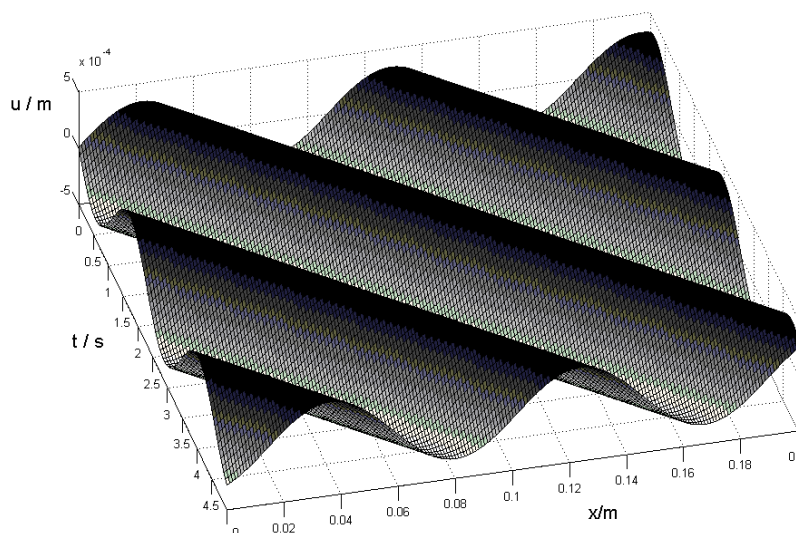
obr. 9.12 Zobrazení výchylky rovinné vlny
