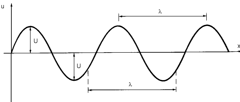
obr. 9.11 Šíření rovinné vlny
