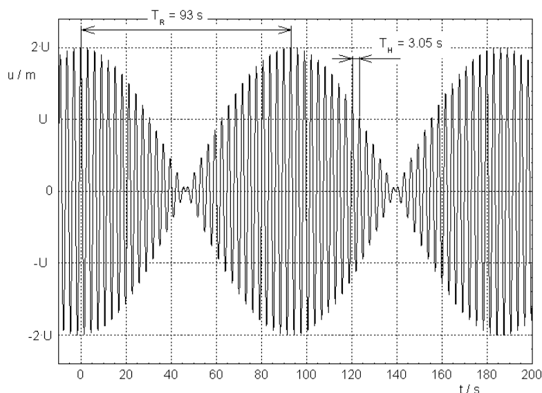
obr. 8.8 Průběh vypočtených rázů
