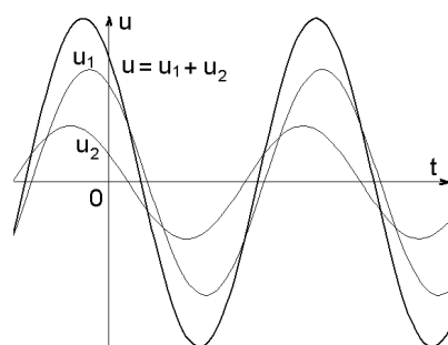
obr. 8.5 Součet dvou harmonických vlnění o stejné frekvenci
