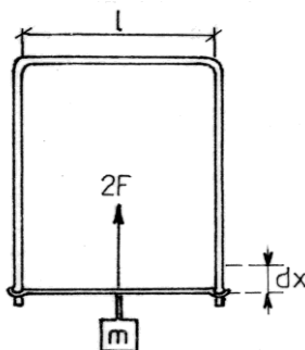
Obr. 2.2 Experimentální určení povrchového napětí
