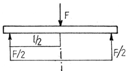
Obr. 1.5 Průhyb nosníku
