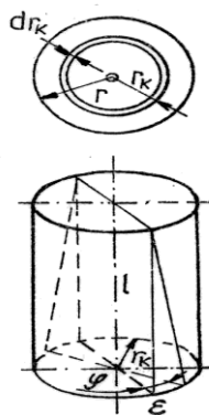
Obr. 1.3 Kroucení tyče
