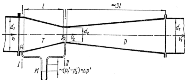
Obr. 4.12 Venturiho trubice
