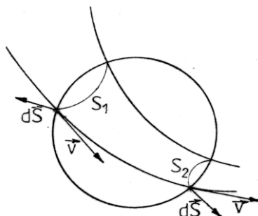
Obr. 4.4 Rovnice kontinuity pro stlačitelné kapaliny
