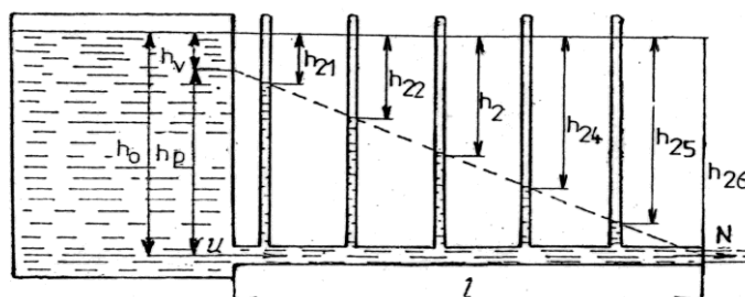
Obr. 4.15 Pokles tlaku způsobený vnitřním třením kapaliny
