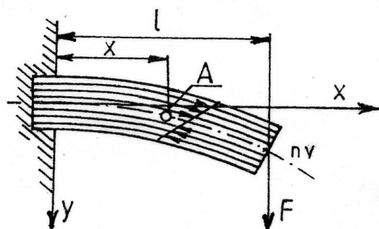
Obr. 1.4 Ohyb krakorce
