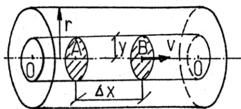
Obr. 4.18 Laminární proudění ve válcovém potrubí
