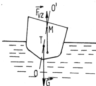
Obr. 3.5 Metacentrum
