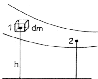
Obr. 4.6 Bernoulliho rovnice
