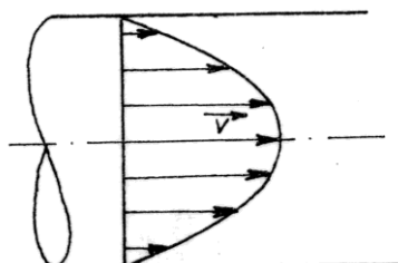
Obr. 4.16 Rozložení rychlostí laminárního proudění ve válcovém potrubí
