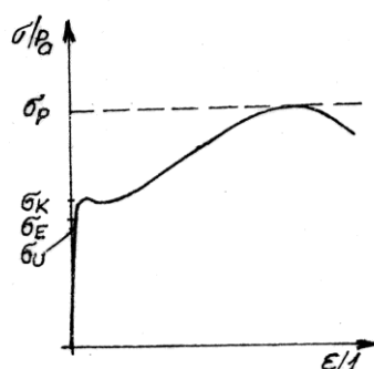
obr.1.1 Závislost napětí na relativním prodloužení
