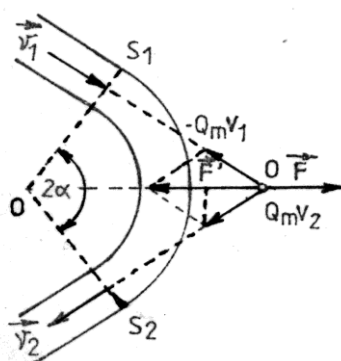
Obr. 4.13 Věta o hybnosti kapalin
