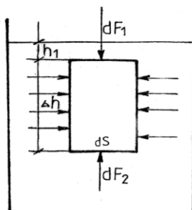
Obr. 3.4 K odvození Archimédova zákona
