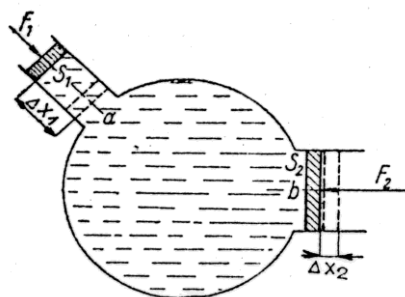
Obr. 3.1 Pascalův zákon
