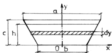
Obr. 3.12 Označení rozměrů hráze
