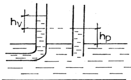
Obr. 4.11 Pitotova trubice
