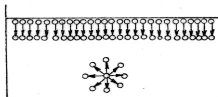
Obr. 2.1 Rozložení sil působících na molekuly v kapalině
