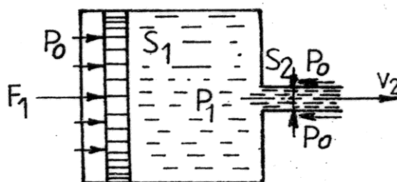
Obr. 4.8 Výtok kapaliny za přetlaku
