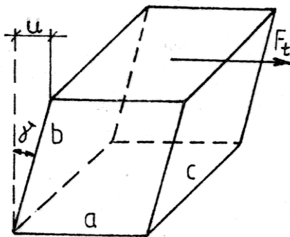
Obr. 1.2 Posunutí způsobené tečnou silou
