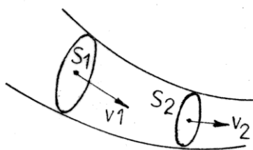
Obr. 4.5 Rovnice kontinuity pro nestlačitelné tekutiny
