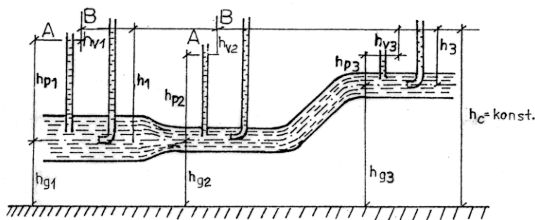
Obr. 4.7 Změny tlaku v potrubí podle Bernoulliovy rovnice
