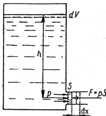
Obr. 3.2 Tlak v kapalině způsobený tíží
