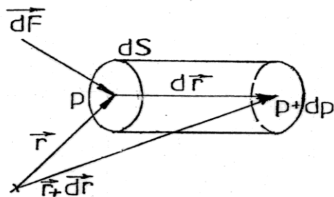
Obr. 3.3 K odvození Eulerovy rovnice
