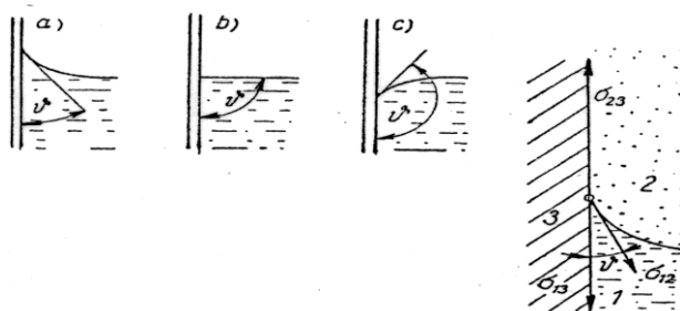
Obr. 2.3 Různé případy chování kapaliny ve styku se stěnou nádoby
