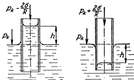
Obr. 2.4 Kapilární elevace a deprese
