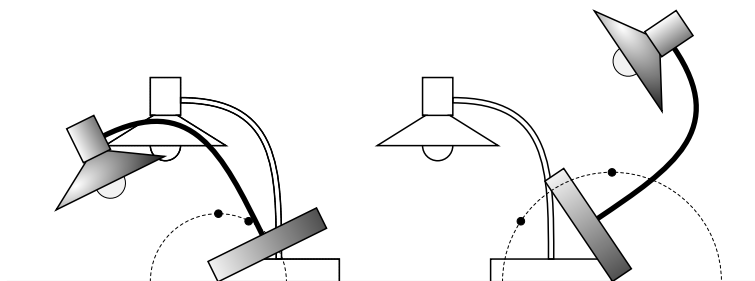
Obrázek 11: Všechny body tělesa (a tedy i těžiště) se při překlápění otáčejí kolem bodu, který je krajním bodem podstavy. Převrnutí tělesa znamená vychýlit jej do takové míry, že se těžiště dostane nad bod otáčení. Jak vidíme na obrázku, lampičku lze na jednu stranu překlopit snáze než na druhou stranu.
