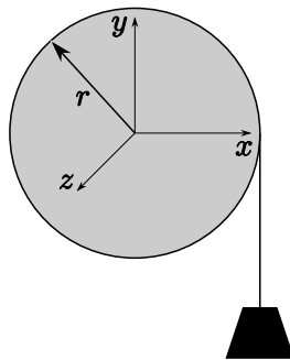
Obrázek 8: Z bubnu se odmotává vlákno, na kterém visí závaží. Existuje tedy vztah mezi úhlovou rychlostí bubnu a rychlostí závaží.
