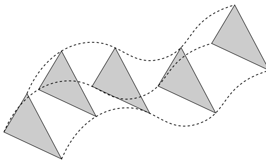
Obrázek 5: Při translačním pohybu tuhého tělesa se jednotlivé částice pohybují po trajektoriích, které jsou stejné jen navzájem posunuté.
