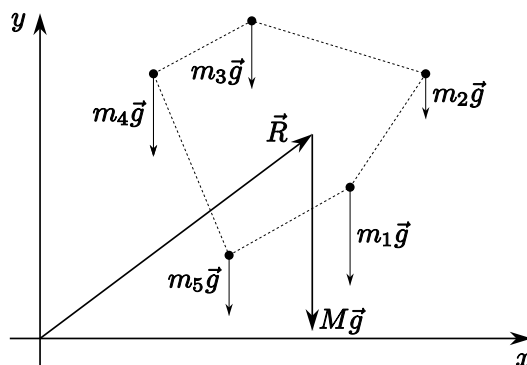
Obrázek 4: Nechtě těleso složeno z několika hmotných bodů. Hledáme takový bod, do kterého lze soustředit hmotnost celého tělesa při zachování stejného momentu gravitační síly.
