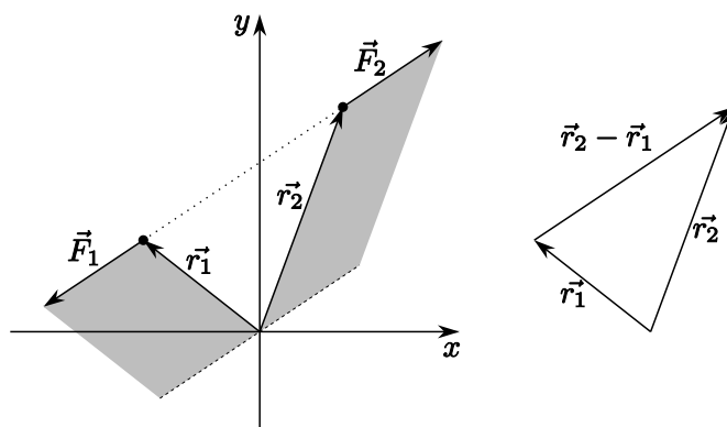
Obrázek 3: Dvě částice na sebe mohou vzájemně působit momentem síly. Oba momenty jsou vždy stejně velké a opačně orientované. Na pravé části obrázku je zakreslen vektor \mathbf{r}_2 - \mathbf{r}_1 , který je rovnoběžný s působícími silami, což využijeme při důkazu.
