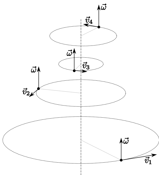
Obrázek 6: Při rotačním pohybu tuhého tělesa se jednotlivé částice pohybují po kružnicích, jejichž osa je společná a nazývá se osa rotace. Úhlová rychlost všech částic je stejná. Je to vektor rovnoběžný s osou rotace.
