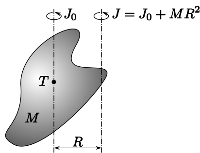
Obrázek 12: Steinerova věta umožňuje snadno vypočítat moment setrvačnosti, jestliže posuneme osu rotace z těžiště o vzdálenost R .
