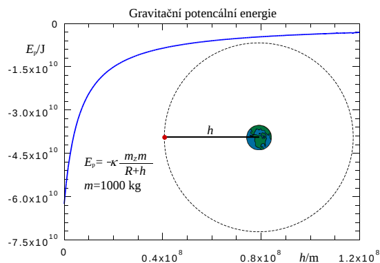
obr. 12 Gravitační potenciální energie vysoko nad Zemí (satelit)
