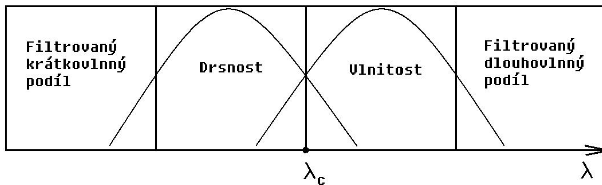
Obr. 3 Oblasti drsnosti a vlnitosti
